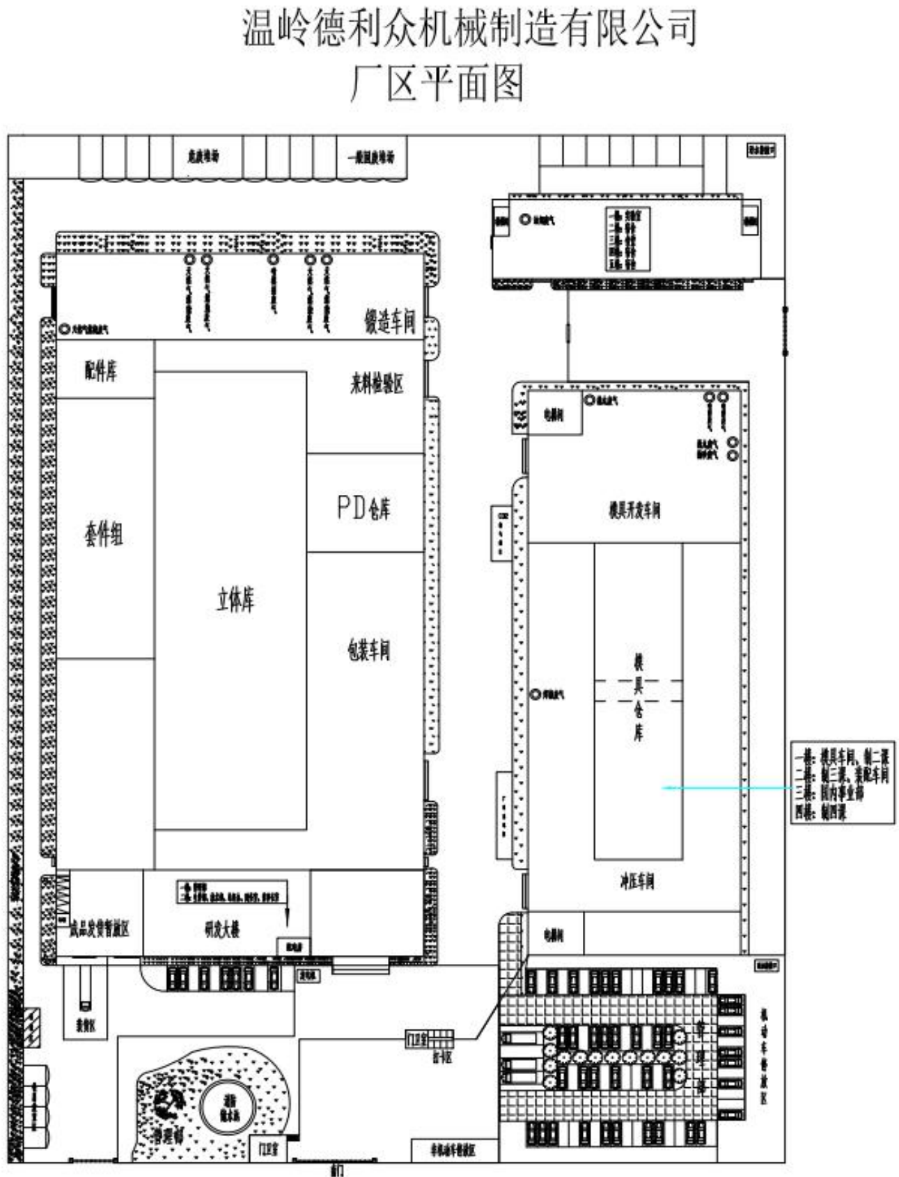
附图 2 厂区总平面布置图
