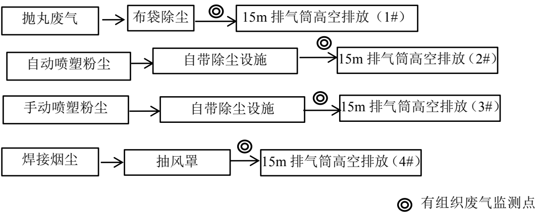
图 6-2 废气监测点位示意图
