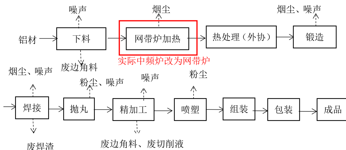
图 2-3 本项目实际生产工艺及产污环节图
