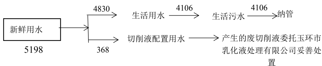
图 2-1 本项目用水平衡图
