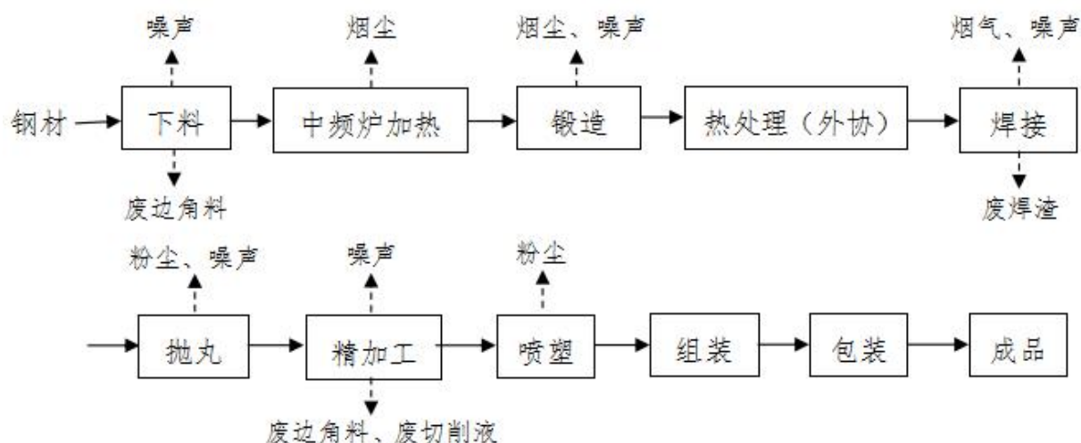
图 2-2 本项目环评生产工艺及产污环节图
